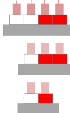
Inkoppling till plinten med 4-, 3- och 2-ledarkabel.
